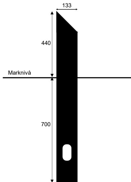
Modell för platsgjutning
